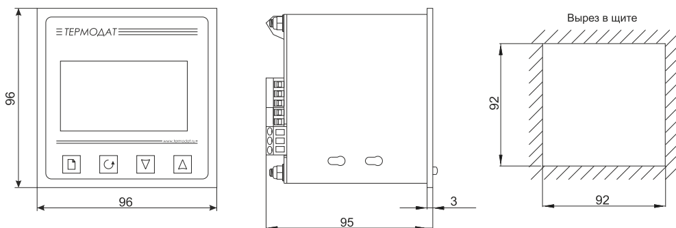
Основной блок
